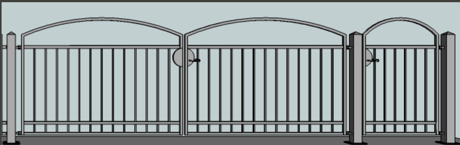
MRK 120 14 / 1+2 korkeus 1200 mm | MRK 150 16 / 1+2 korkeus 1500 mm
