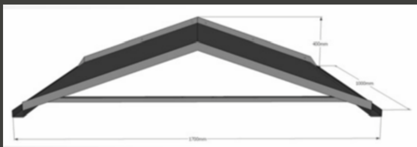
harjakatos
